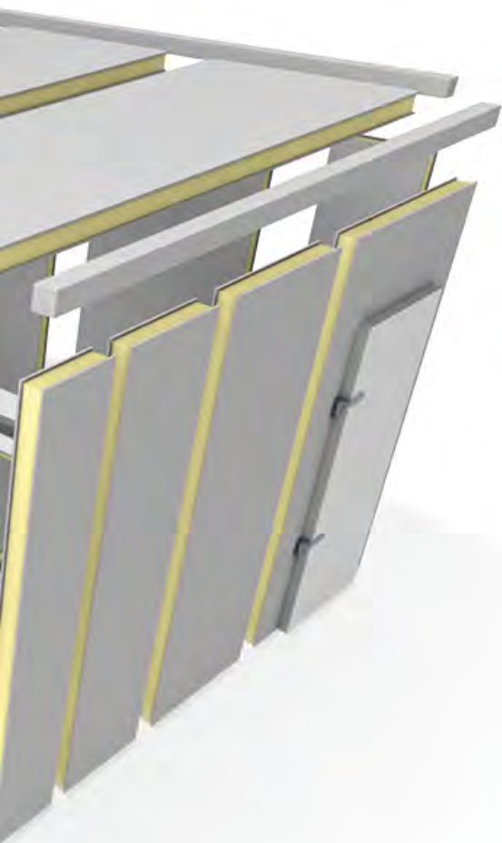
跨墙式安装
